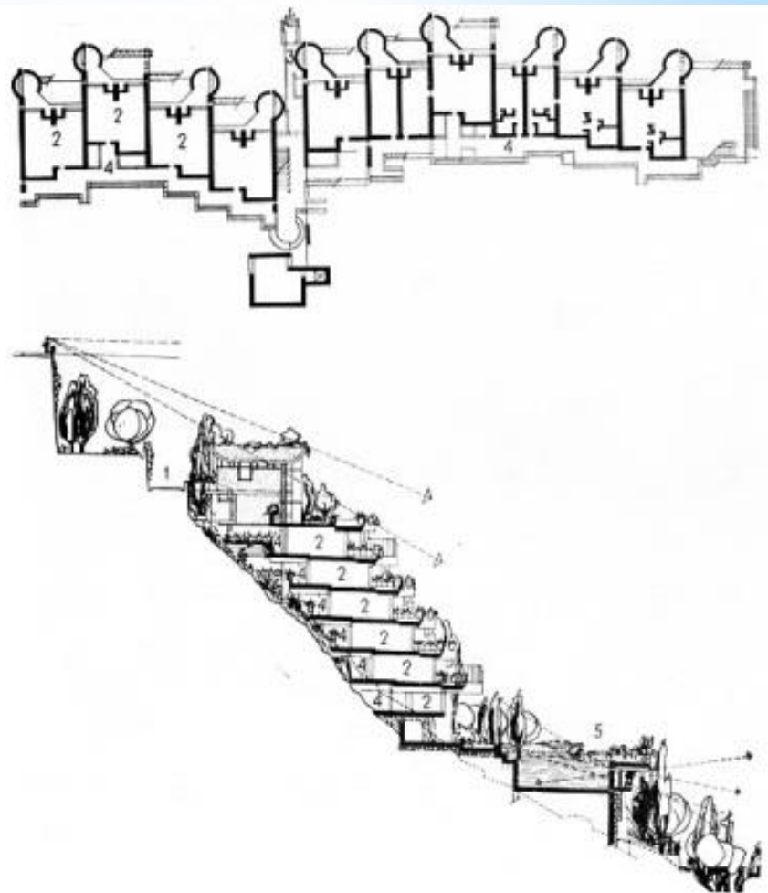
Рис. 74. Отель «Монте-Тауро» в Таормино, Сицилия (архит. А. Гатти). Общий вид с моря, план одного из жилых этажей, поперечный разрез 1 — вход в отель; 2 — номер; 3 — проход к лифтам; 4 — общие галереи; 5 — бассейн
