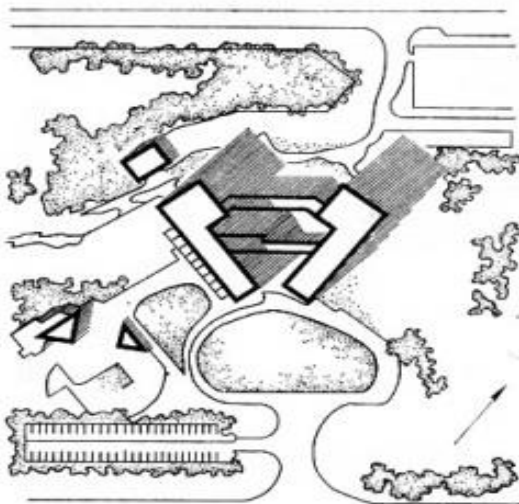
Рис. 75. Отель «Де-Ла-Пе» в Того (архит. Шепс). Общий вид, генплан
